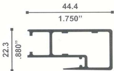
*9955 TRASLAPE PUERTA 0.503 Kg./m
