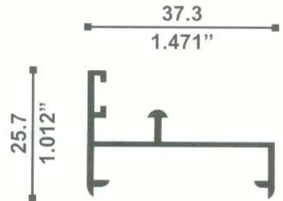
11838 RIEL 0.250 Kg./m
