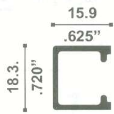
7525 CERCO FIJO ECONOMICO 0.224 Kg./m
