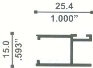
11836 CERCO TRASLAPE 0.166 Kg./m
