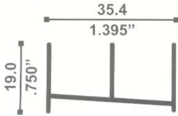
11387 RIEL INFERIOR 0.233 Kg./m
