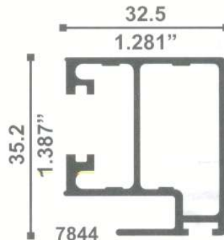
7844 CERCO TRASLAPE VENTANA 0.627 Kg./m
