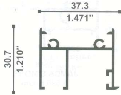
11835 JAMBA Y CABEZAL 0.357 Kg./m
