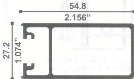
* 7847 CERCO CHAPA 3.445 kg./m
