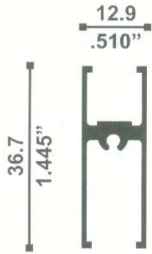
11837 CABEZAL Y ZOCLO 0.246 Kg./m
