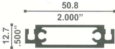
7101 INTERMEDIO MOSQUITERO 0.584 Kg./m
