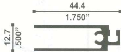
6533 CERCO MOSQUITERO HORIZONTAL 0.378 Kg./m
