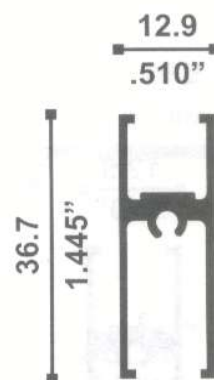
11837 CABEZAL Y ZOCLO 0.246 Kg./m
