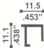
7014 JUNQUILLO 0.101 Kg./m
