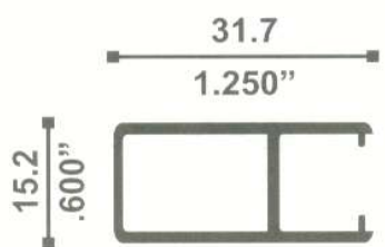
8320 CERCO VENTANA 0.319 Kg./m
