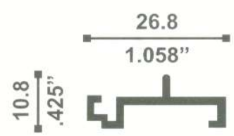
9966 ADAPTADOR MOSQUITERO 0.176 Kg./m
