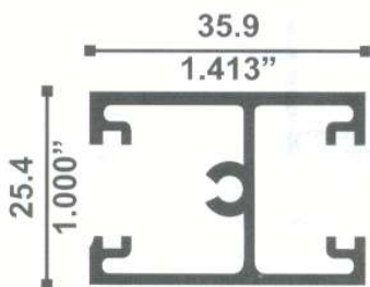
9082 INTERMEDIO 0.612 Kg./m
