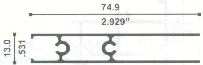
7825 ZOCLO PUERTA 0.695 Kg./m
