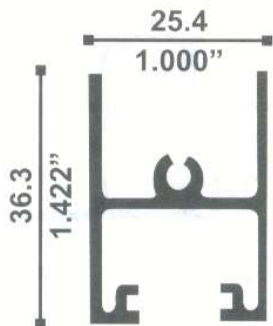
7836 CABEZAL 0.482 Kg./m
