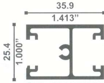
9082 INTERMEDIO 0.591 Kg./m
