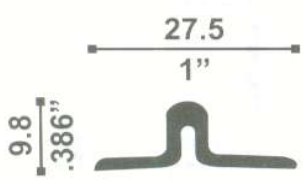
7818 RIEL ADICIONAL 0.191 Kg./m
