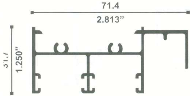
7819 JAMBA CON MOSQUITERO 0.780 Kg./m
