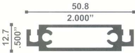
7101 INTERMEDIO MOSQUITERO 0.584 Kg./m
