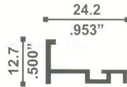
7013 PORTA VIDRIO 0.163 Kg./m
