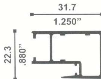
9954 TRASLAPE VENTANA 0.430 Kg./m
