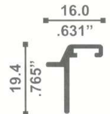
10220 ADAPTADOR OXXO 0.134 Kg./m
