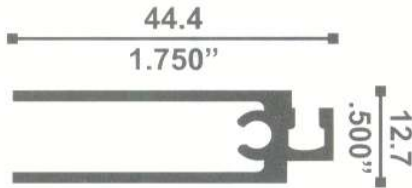
6533 CERCO MOSQUITERO HORIZONTAL 0.378 Kg./m
