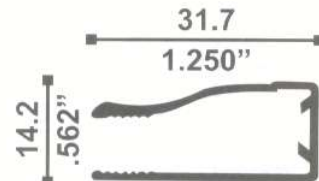
9525 MARCO 1 1/4'' 0.254 Kg./m
