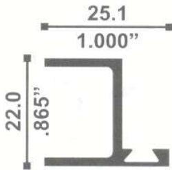
7102 BATIENTE STD. 0.327 kg./m
