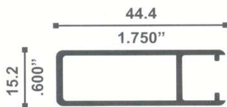
*7821 CERCO PUERTA 0.380 Kg./m
