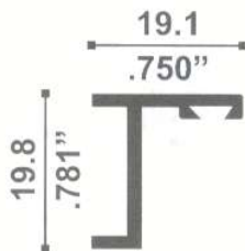
4127 BATIENTE 0.186 Kg./m
