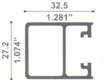
7843 CERCO JALADERA VENTANA 0.576 Kg./m
